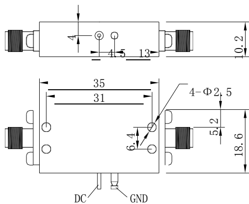
UNIT:mm XB-02A
